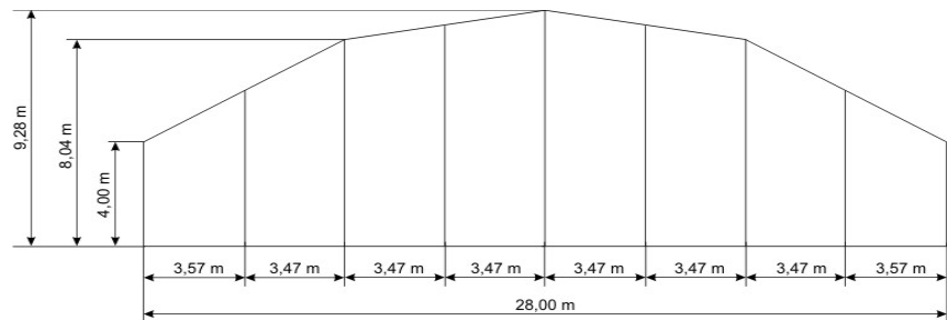
Вертикальный разрез конструкции
