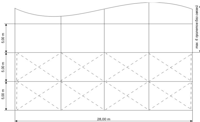
План конструкции
