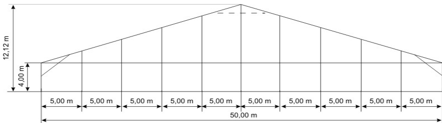
Вертикальный разрез конструкции
