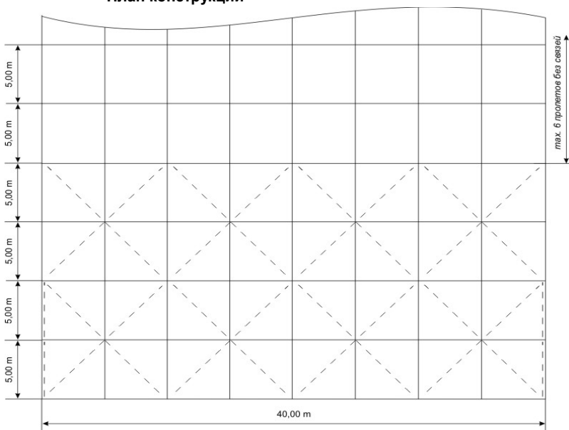
План конструкции
