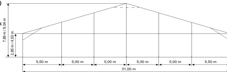
Вертикальный разрез конструкции
