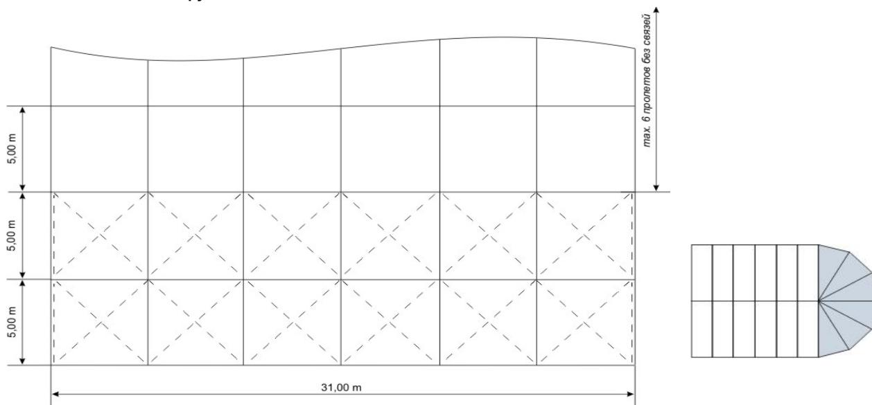
План конструкции
