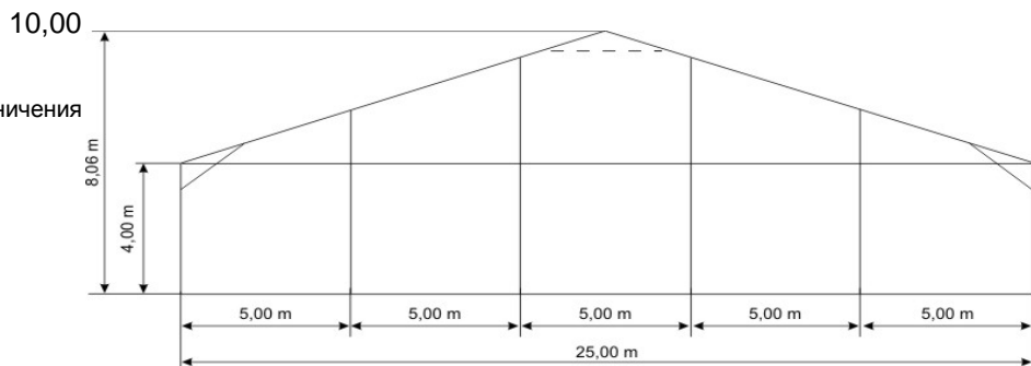
Вертикальный разрез конструкции
