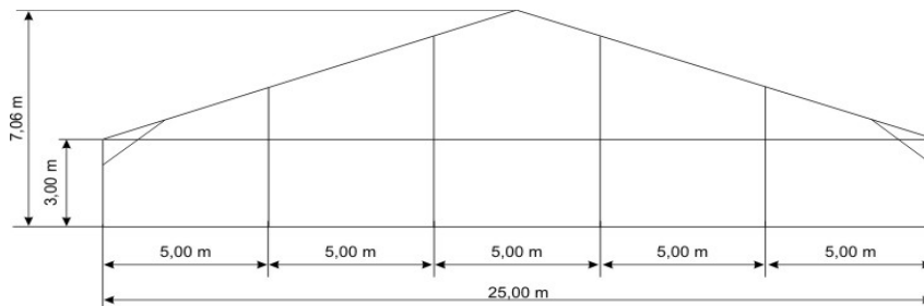
Вертикальный разрез конструкции
