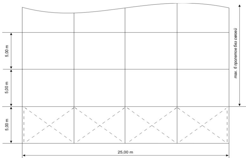
План конструкции
