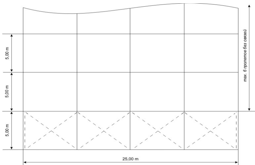
План конструкции
