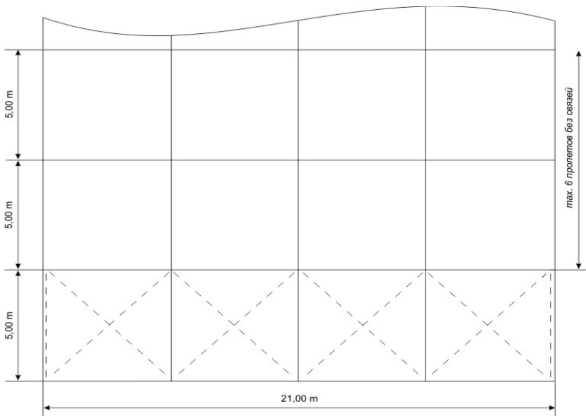
План конструкции
