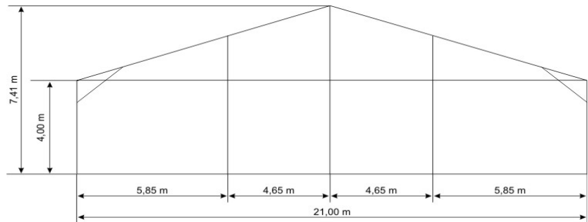
Вертикальный разрез конструкции
