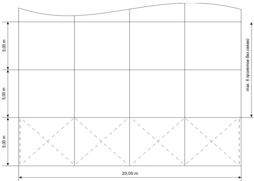
План конструкции
