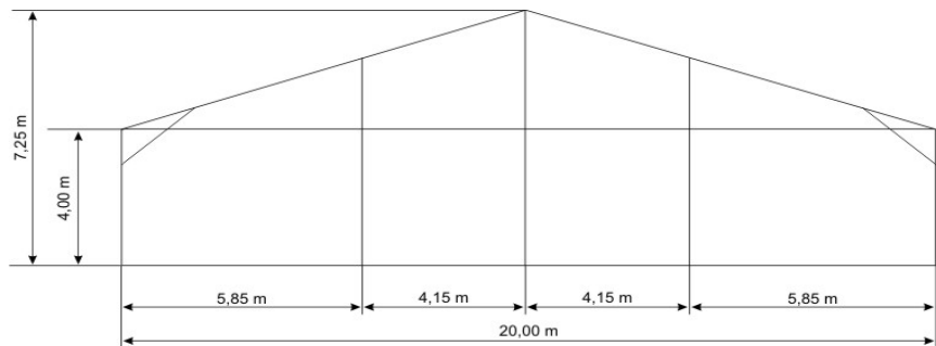
Вертикальный разрез конструкции
