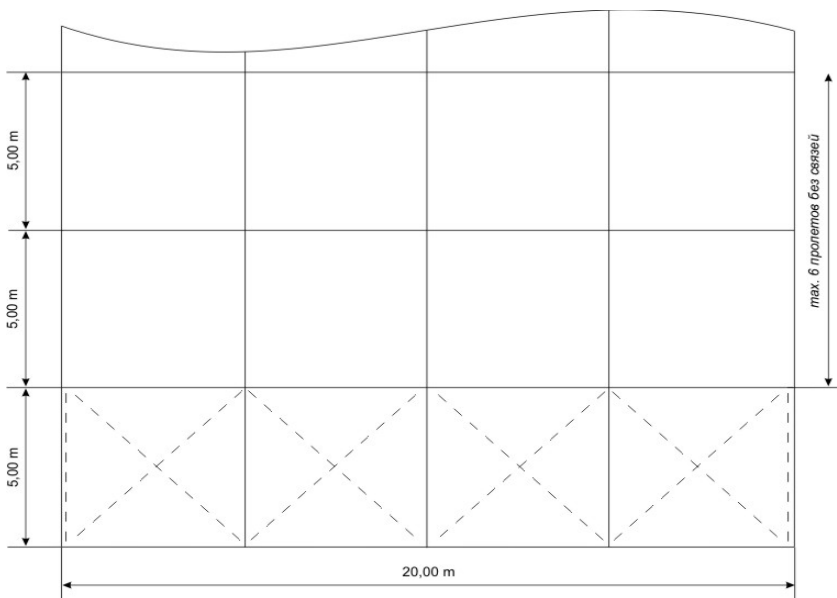
План конструкции
