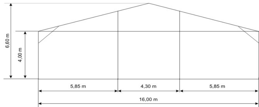
Вертикальный разрез конструкции
