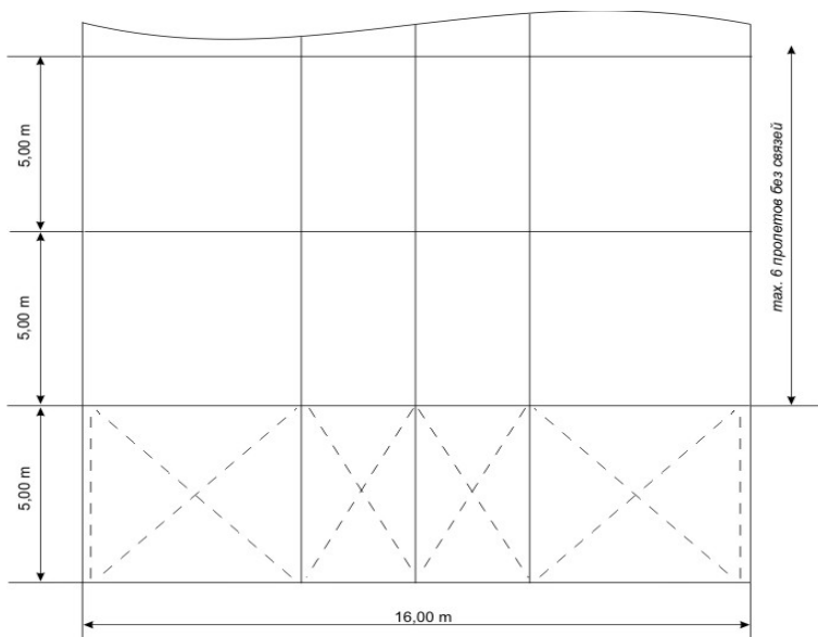
План конструкции
