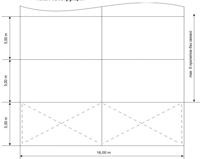
План конструкции
