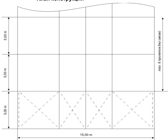
План конструкции
