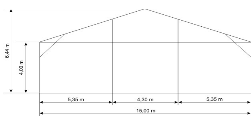
Вертикальный разрез конструкции
