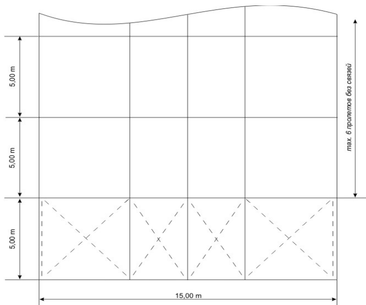
План конструкции
