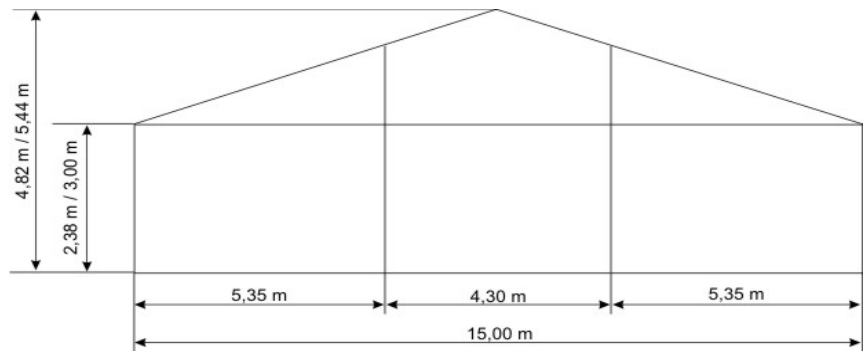
Вертикальный разрез конструкции
