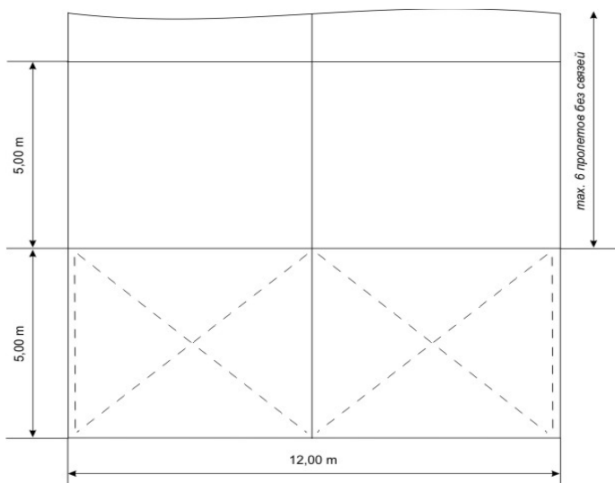
План конструкции
