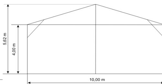
Вертикальный разрез конструкции
