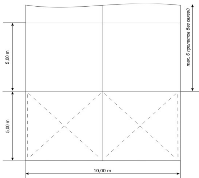
План конструкции
