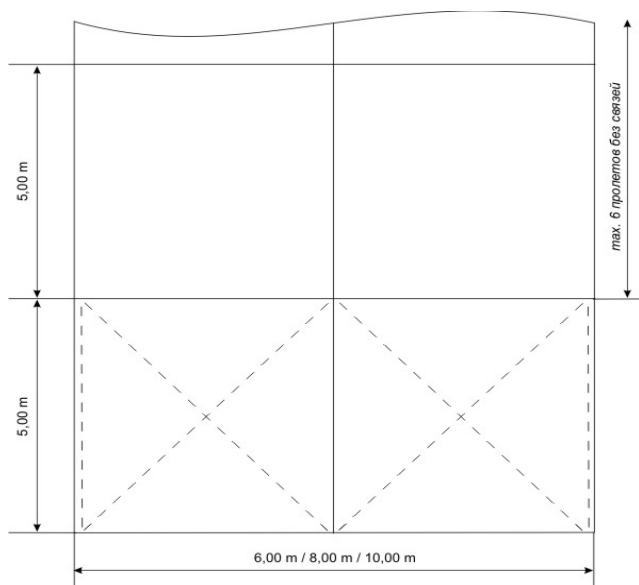
План конструкции
