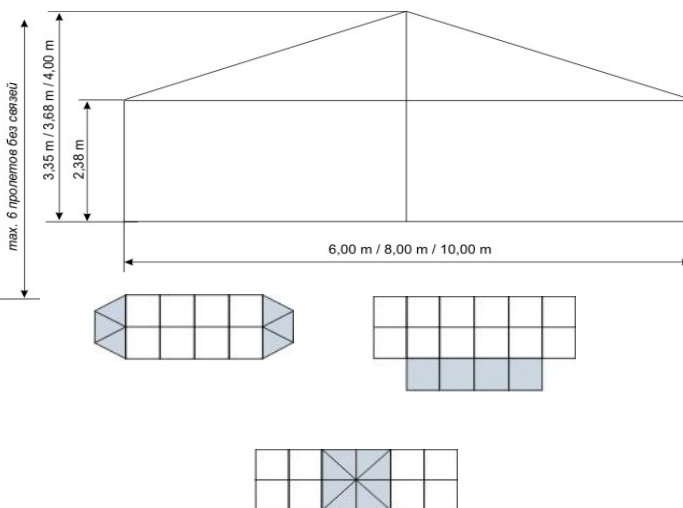
Вертикальный разрез конструкции
