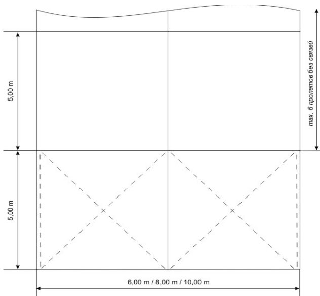
План конструкции
