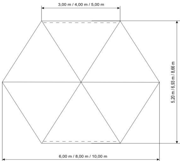
План конструкции
