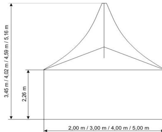
Вертикальный разрез конструкции
