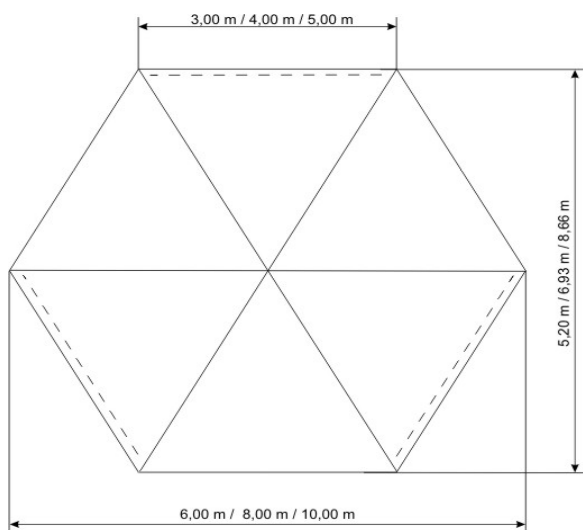
План конструкции
