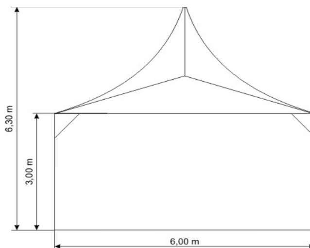
Вертикальный разрез конструкции
