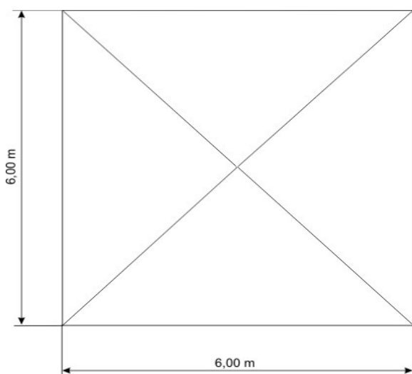
План конструкции
