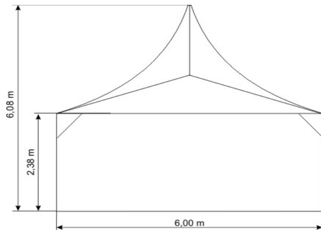
Вертикальный разрез конструкции
