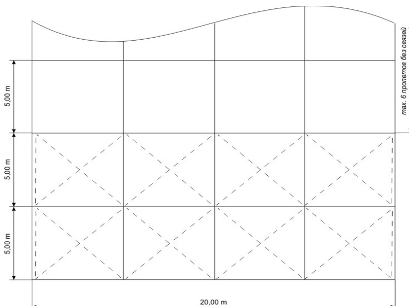
План конструкции
