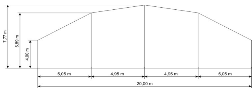
Вертикальный разрез конструкции
