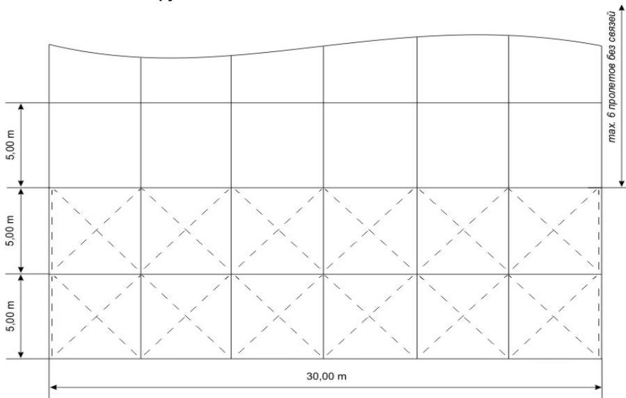
План конструкции
