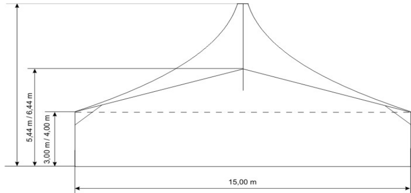
Вертикальный разрез конструкции
