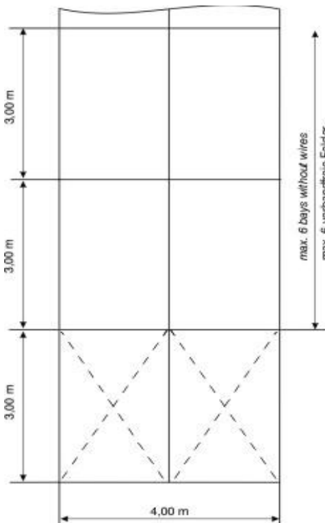
План конструкции
